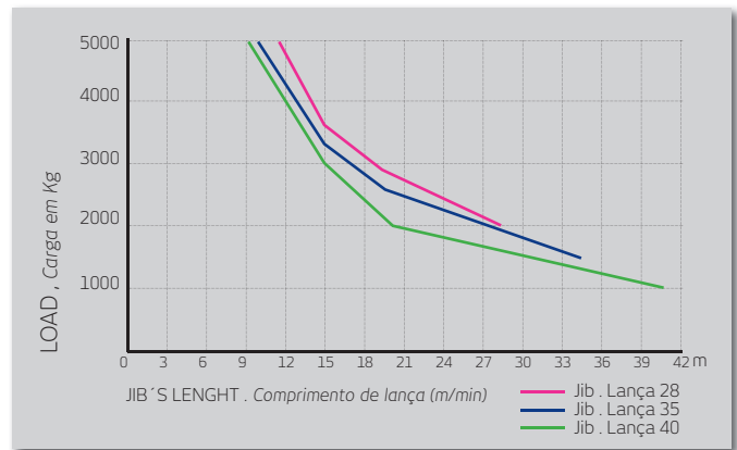
LOAD DIAGRAM DIAGRAMA DE CARGAS
