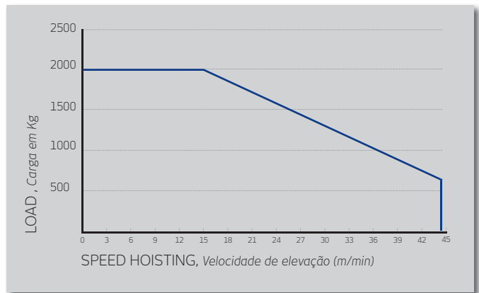
SPEED DIAGRAM DIAGRAMA DE VELOCIDADE
